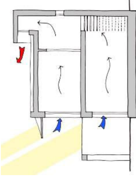
Fig.3.9 - Stratégie d'éclairage / ventilation en été
