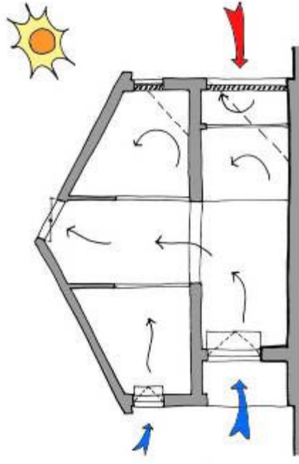
Fig. 3.3 - Été : stratégie de ventilation
