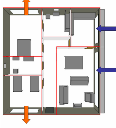
Fig.3.16 - Stratégie de ventilation d'été
