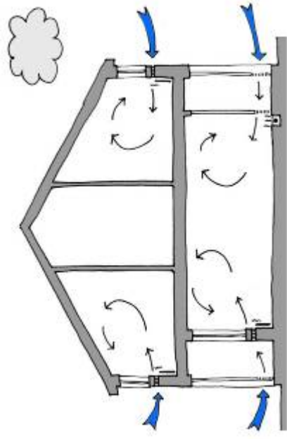
Fig. 3.4 - Hiver : stratégie de ventilation pendant la journée
