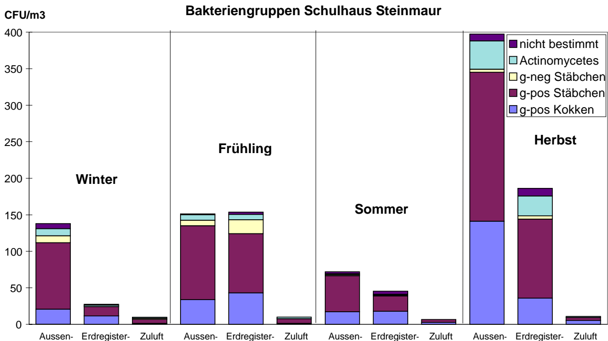
Abb. 23: Bakterien in der Aussen-, der Erdregister- und der Zuluft in der Anlage Schulhaus Steinmaur
