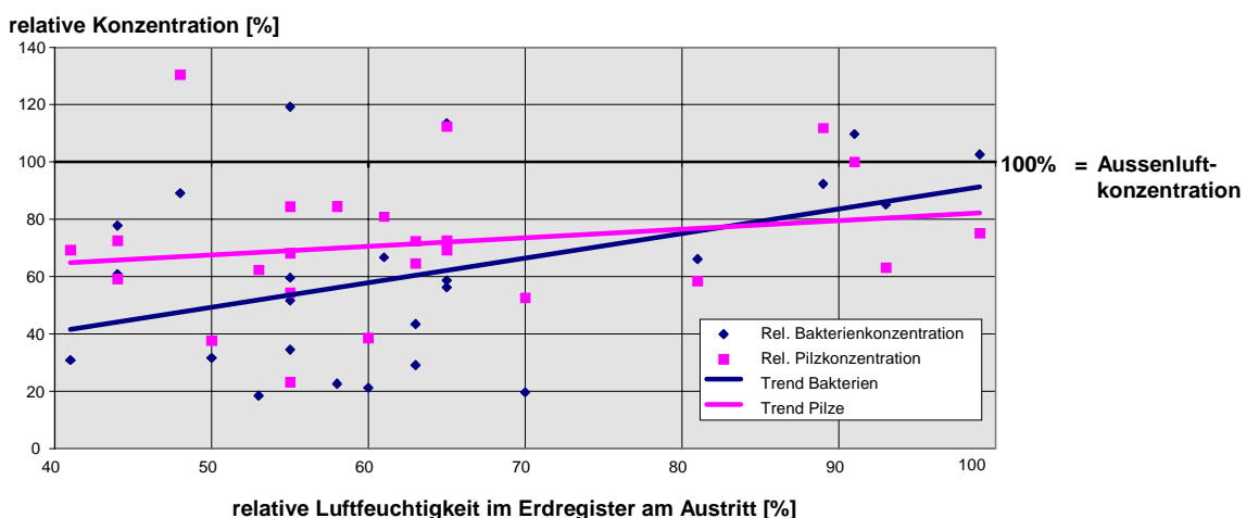
Abb. 25: Relative Veränderung der Konzentrationen der Bakterien bzw. Pilze im Erdregister im Vergleich zur Konzentration in der Aussenluft (=100%) in Abhängigkeit von der relativen Luftfeuchtigkeit im Erdregister. Korrelation der relativen Differenz der Bakterien mit Luftfeuchtigkeit 0,43 (95%-Signifikanzniveau: 0,39). Die Abhängigkeit der Pilze zu der relativen Luftfeuchtigkeit korreliert nicht signifikant.
